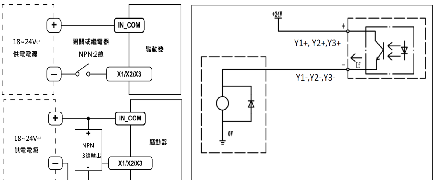
輸入迴路
