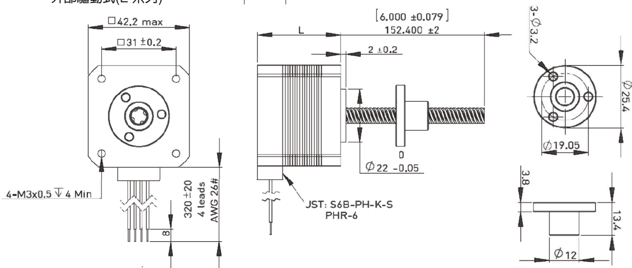
外部驅動式(E 系列)
