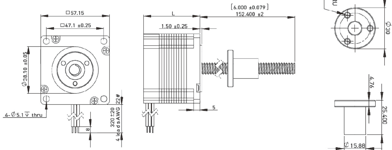
外部驅動式(E 系列)
