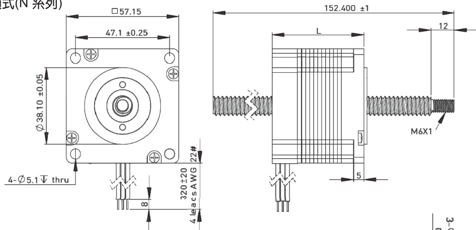
貫通式(N 系列)
