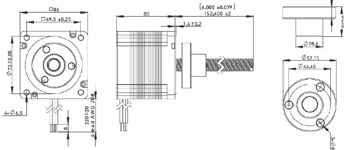
外部驅動式(E 系列)
