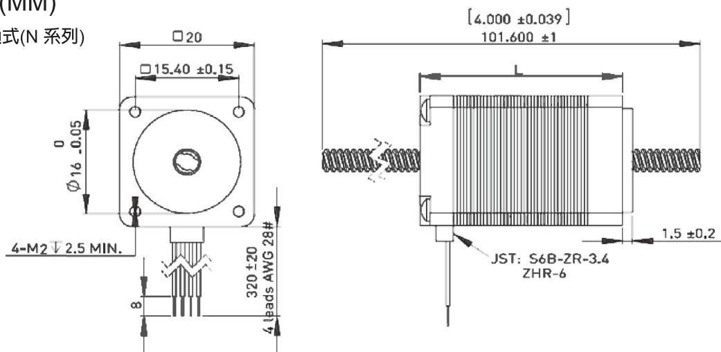
外部驅動式(E 系列)
